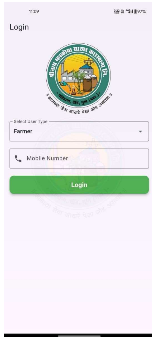
Fig. 8.2. Login Page
